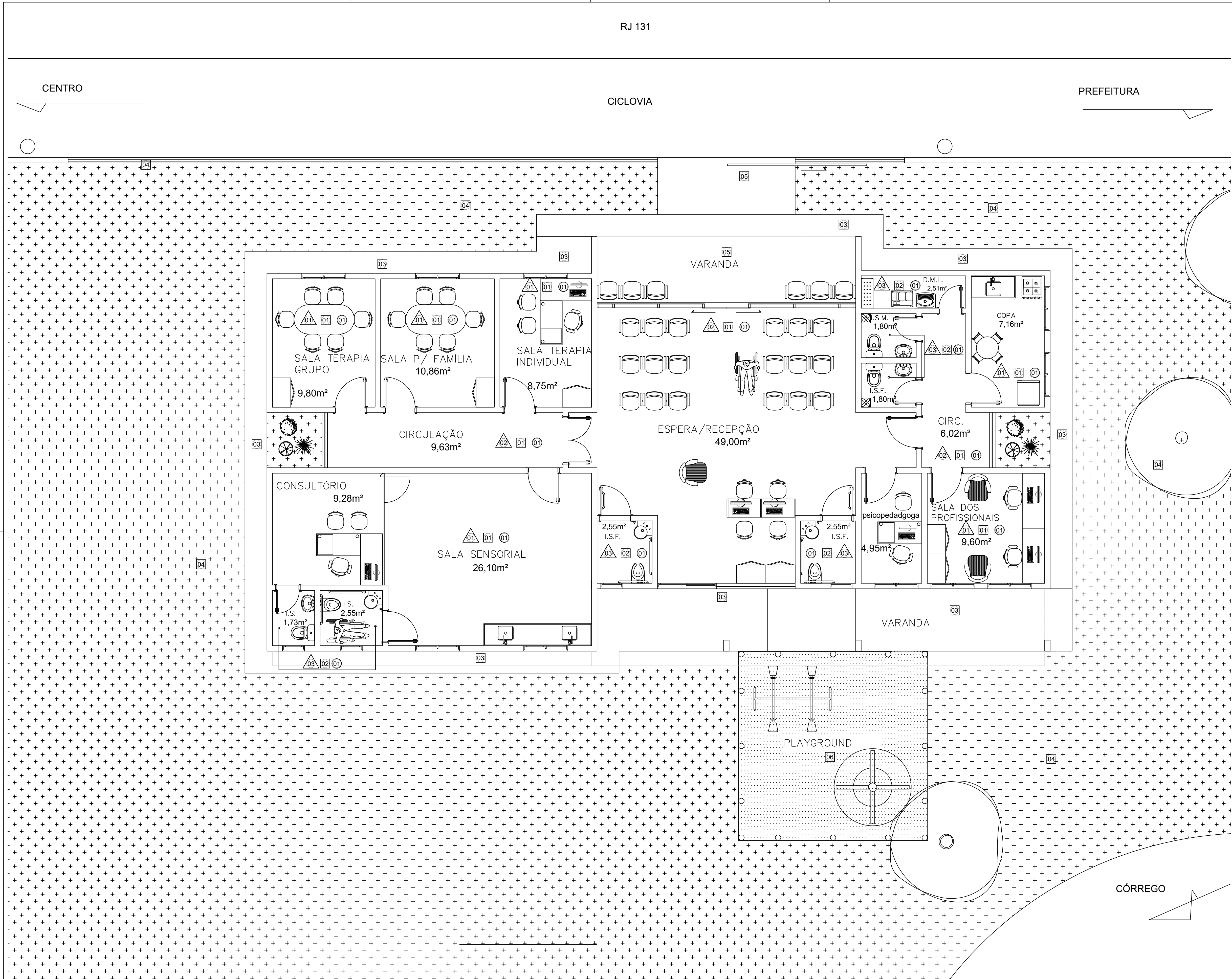
PLANTA DE LAYOUT esc. 1/50
