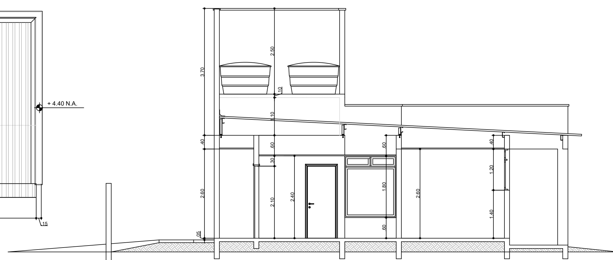
CORTE C-C esc. 1/50
