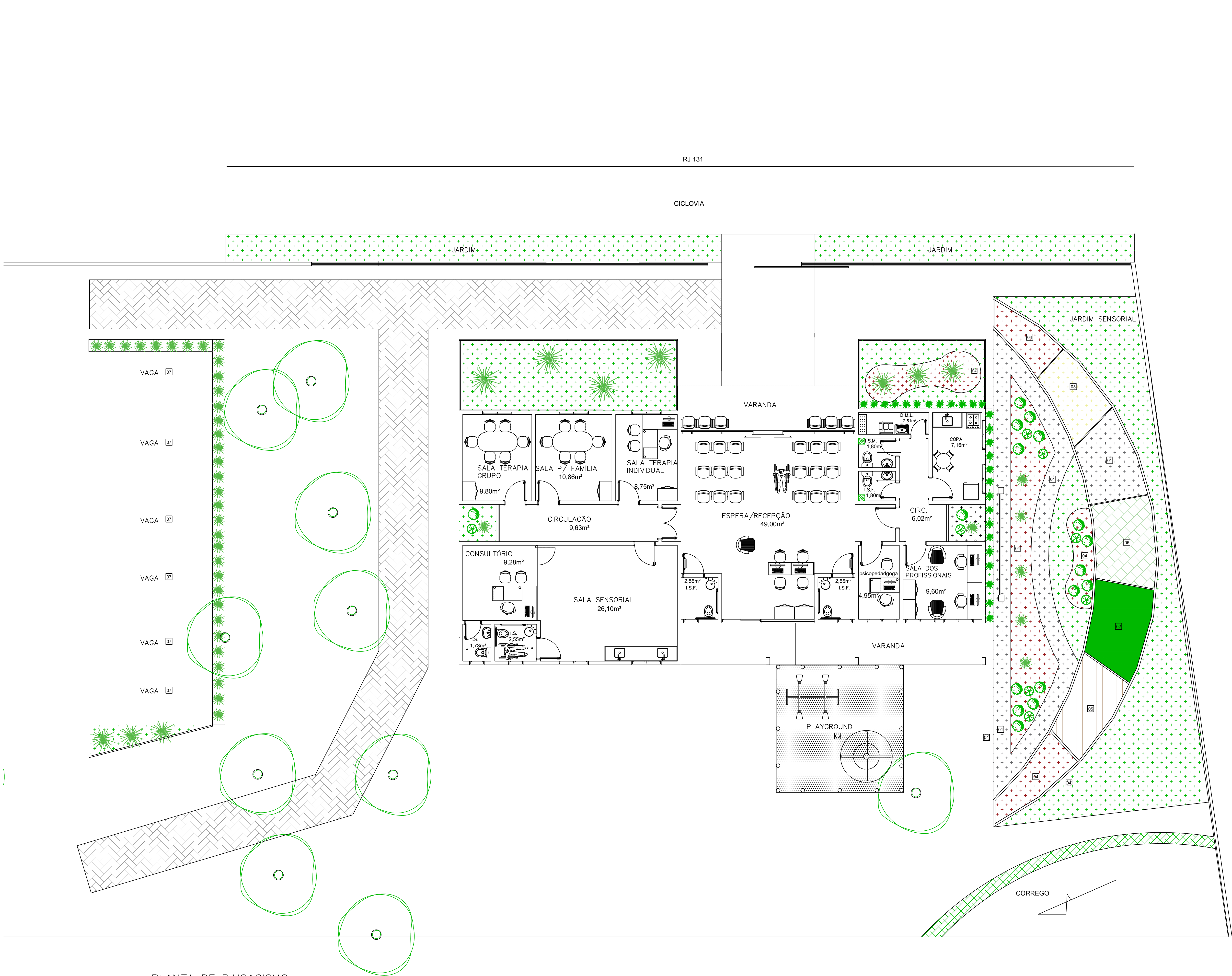
PLANTA DE PAISAGISMO esc. 1/75
